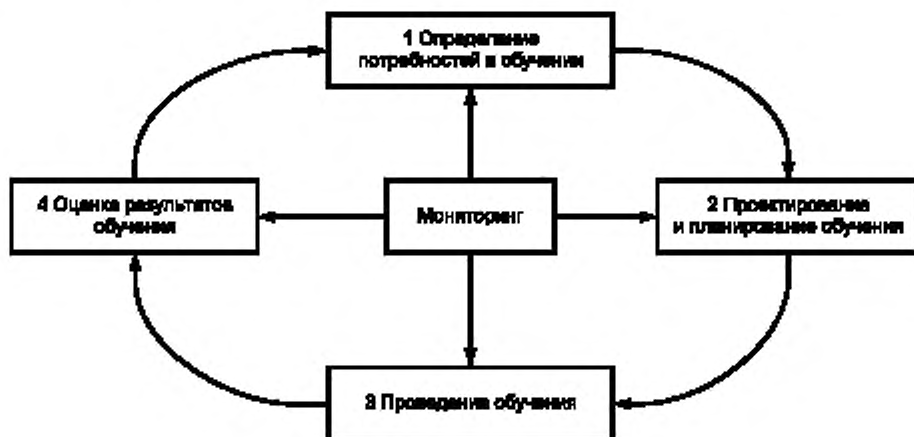
Рисунок 2 — Цикл обучения
