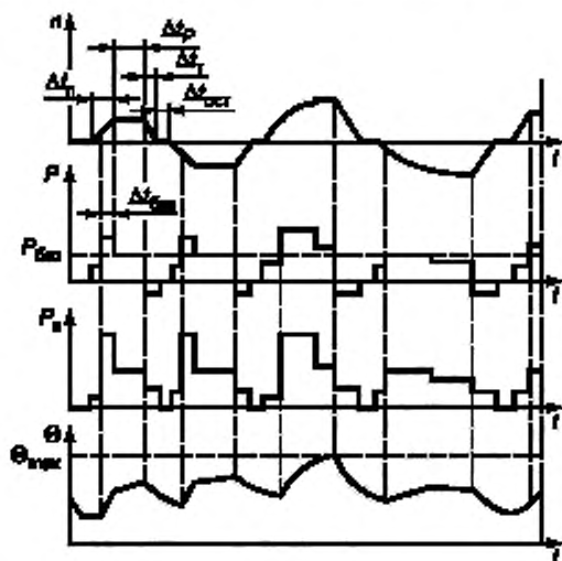
P — нагрузка; P_{\text{баз}} — базовая нагрузка; P_e — электрические потери; \theta — температура; \theta_{\text{max}} — достигнутая максимальная температура; t — время; \Delta t_p — время работы с постоянной нагрузкой; \Delta t_r — время пуска (разгона); \Delta t_e — время электрического торможения; \Delta t_{\text{ост}} — время остановки или отключения питания машин; \Delta t_{\text{баз}} — время работы с базовой нагрузкой; n — частота вращения
