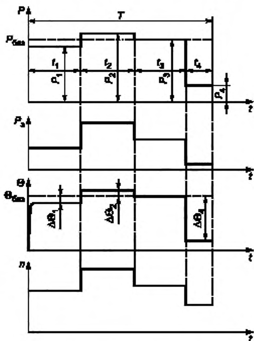
P — нагрузка, P_{\text{баз}} — базовая нагрузка в соответствии с типовым режимом S1, P_{1,2,3,4} — постоянная часть нагрузки внутри одного цикла нагрузки; P_3 — электрические потери, \theta — температура, \theta_{\text{баз}} — температура при базовой нагрузке P_{\text{баз}} ; t — время, t_{1,2,3,4} — время работы с постоянной нагрузкой внутри цикла нагрузки; T — время одного цикла нагрузки, \Delta\theta_{1,2,3} — разница между превышением температуры обмоток при каждой из различных нагрузок внутри одного цикла и превышением температуры при базовой нагрузке в режиме S1; n — частота вращения
