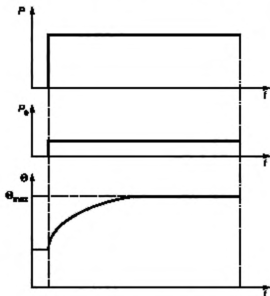
P — нагрузка, P_e — электрические потери; \theta — температура. \theta_{max} — достигнутая максимальная температура. t — время
