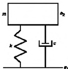
Рисунок А.1 — Система с одной степенью свободы
