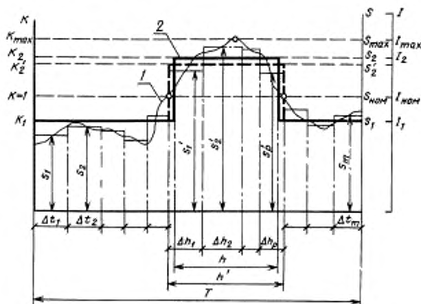
1 — исходный график нагрузки; 2 — двухступенчатый прямоугольный график нагрузки
