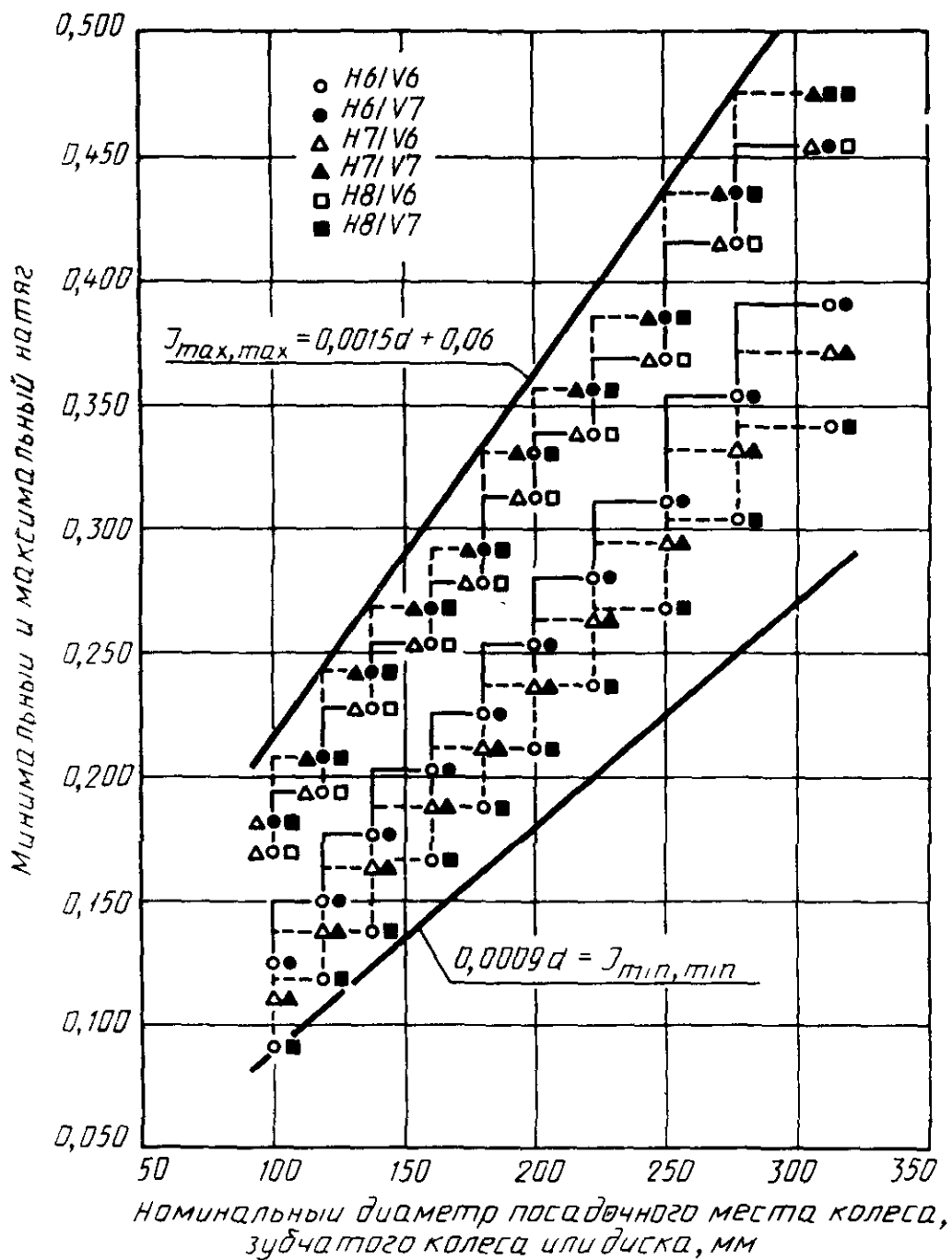
Натяг в соединениях диаметром 100 и 300 мм
