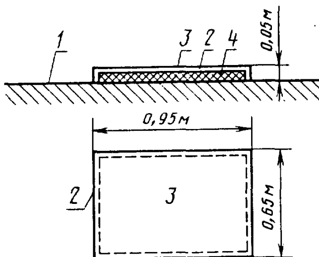
1 – стена; 2 – деревянная рама; 3 – фанера; 4 – стекловата или минераловата
