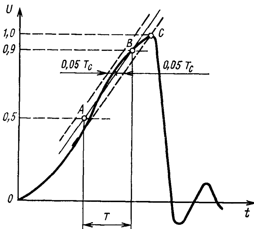
Импульс с линейным фронтом
