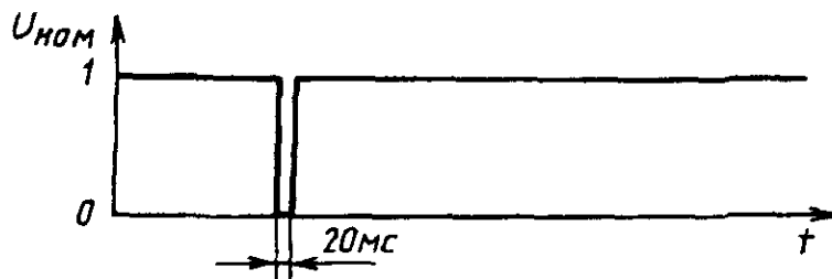
Рисунок 2 — Прерывания напряжения \Delta U=100\% , 20 мс
