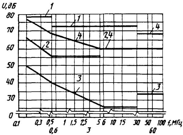
Нормы напряжения радиопомех
