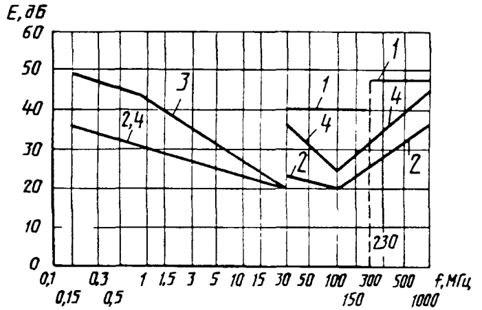
Нормы напряженности поля радиопомех
