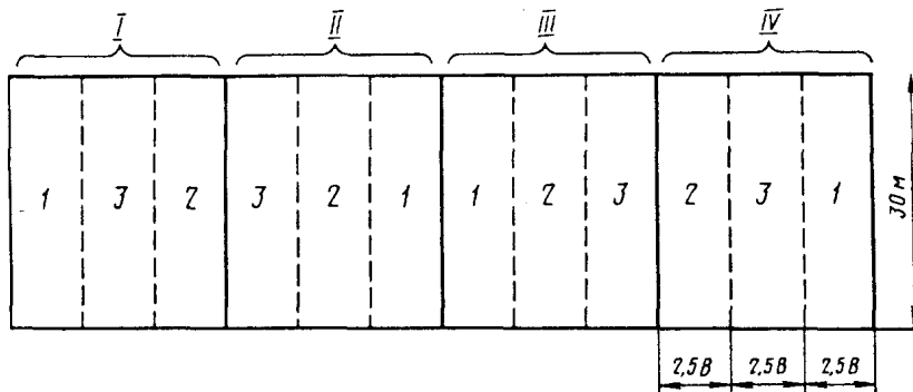
Схема организации участка испытаний
