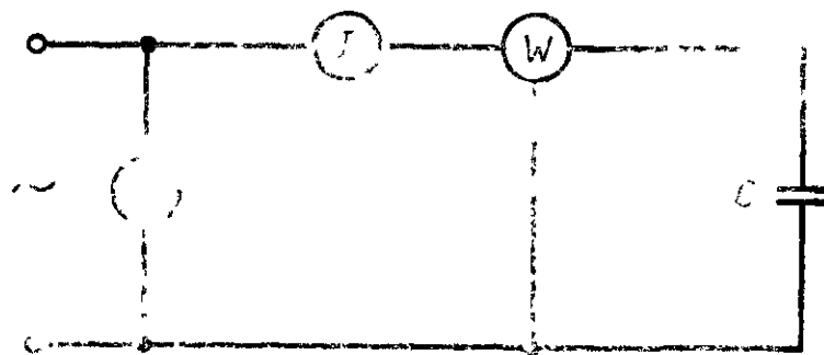
V — вольтметр; I — амперметр, W — ваттметр, рассчитанный на точную работу при \cos\varphi = 0,1 ; C — испытуемый конденсатор
