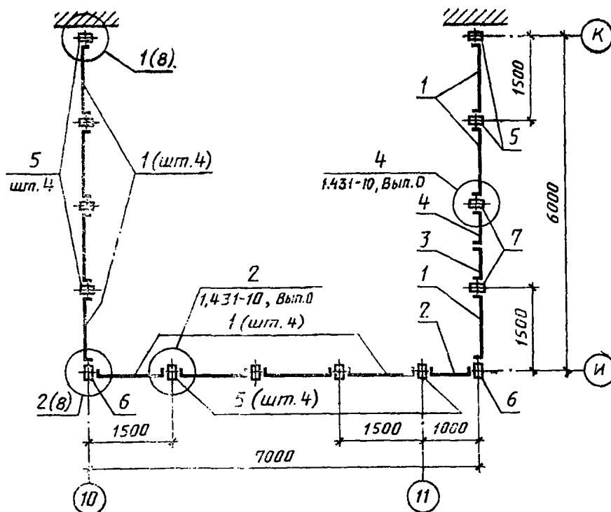
Пример выполнения схемы расположения элементов сборных перегородок
