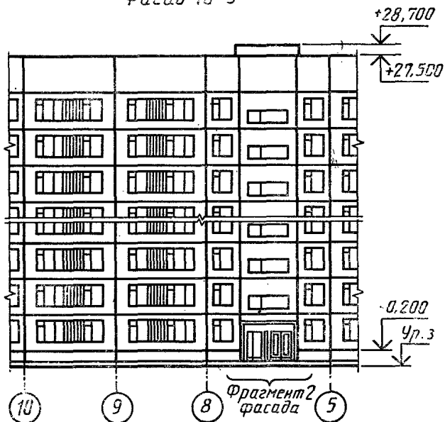
Фасад 10-5
