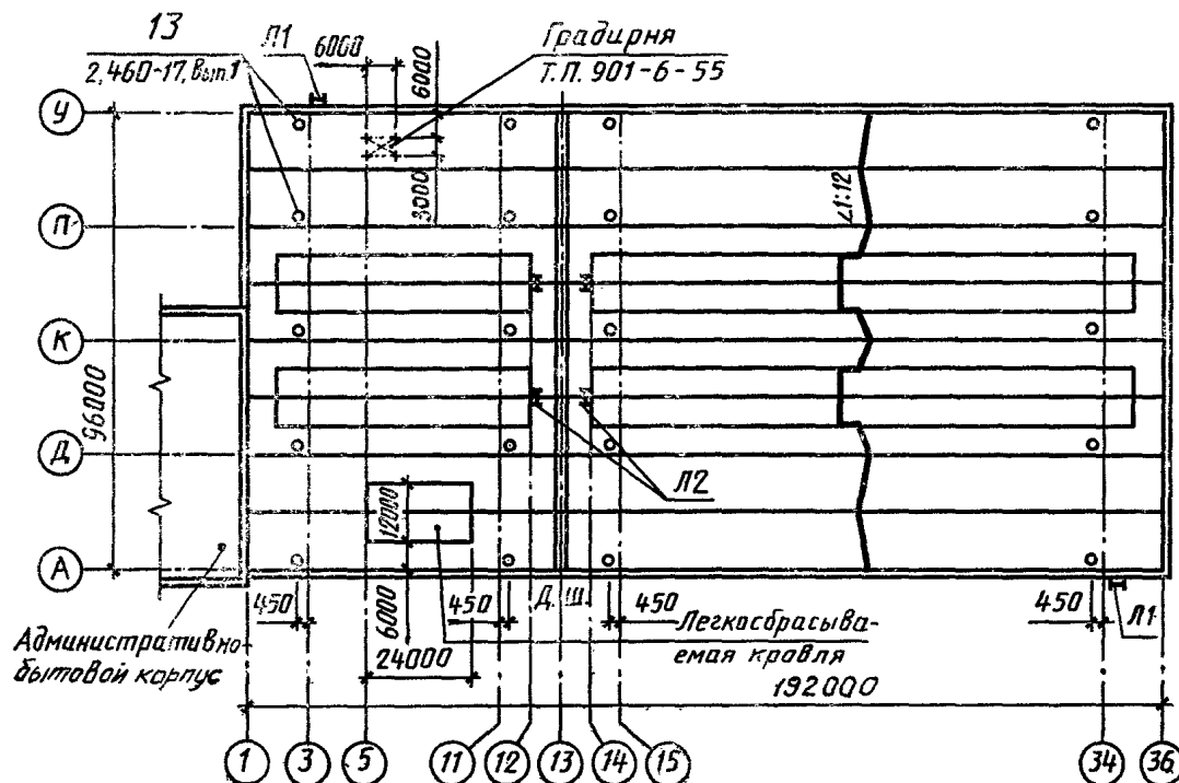
Пример выполнения плана кровли
