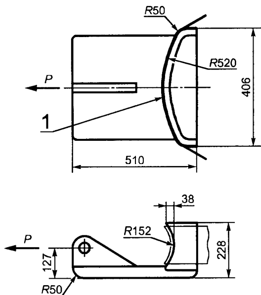
1 — пористый материал, покрытый полотном, толщина 25 мм; P — испытательная нагрузка
