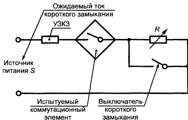
Рисунок Н 3 — Испытание на короткое замыкание
