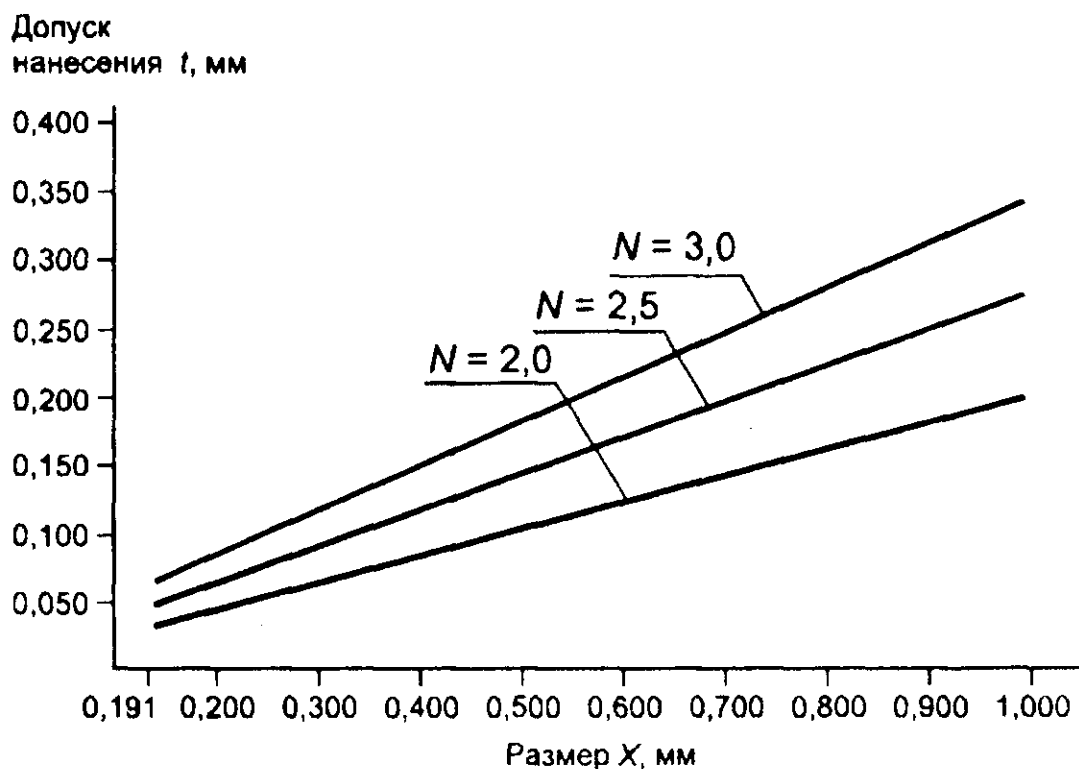
Рисунок 2 — Допуски для «Кода 39»
