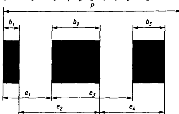
Рисунок 6 — Размеры для декодирования
