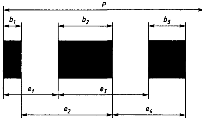
Рисунок 4 — Размеры для допусков
