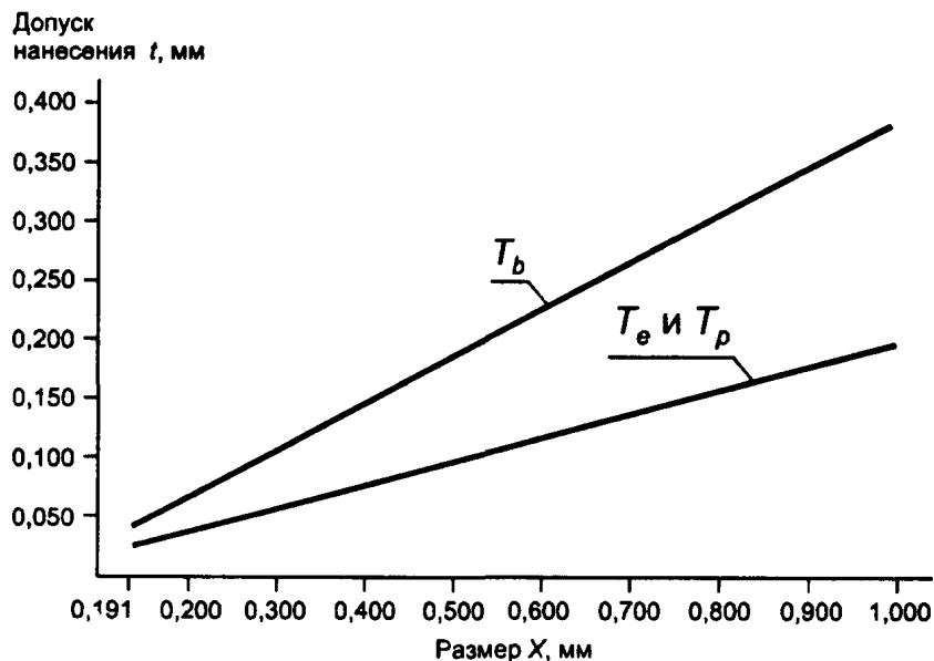
Рисунок 5 — Допуски для «Кода 128»
