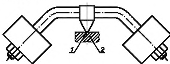
1 — сфера R = 2,5 \text{ мм} ; 2 — образец
