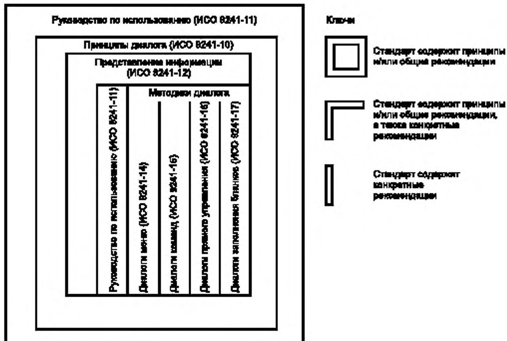
Рисунок А.1 — Соотношение частей программного обеспечения ИСО 9241
