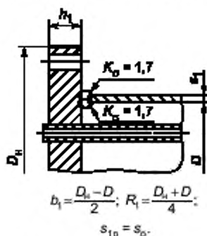
Рисунок 7 — решетка, приваренная втавр к обечайке кожуха
