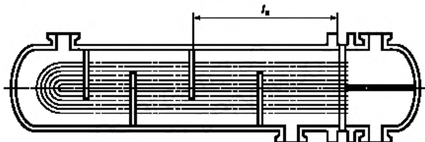
Рисунок 4 — Аппарат с U-образными трубами
