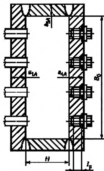
Рисунок 21 — Сварная камера без перегородок
