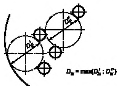
Рисунок 14 — Диаметр окружности, вписанной в максимальную беструбную площадь
