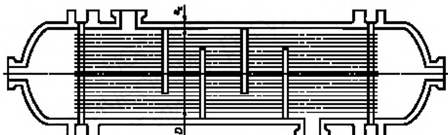
Рисунок 1 — Аппарат с неподвижными трубными решетками
