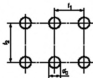
Рисунок Ж.1 — Расположение отверстий по вершинам прямоугольников
