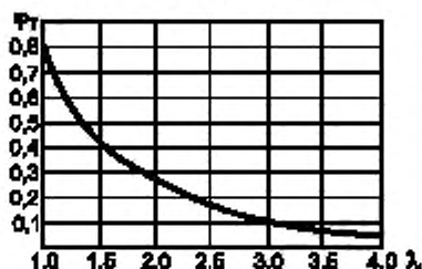
Рисунок 11 — коэффициент уменьшения допускаемого напряжения при продольном изгибе
