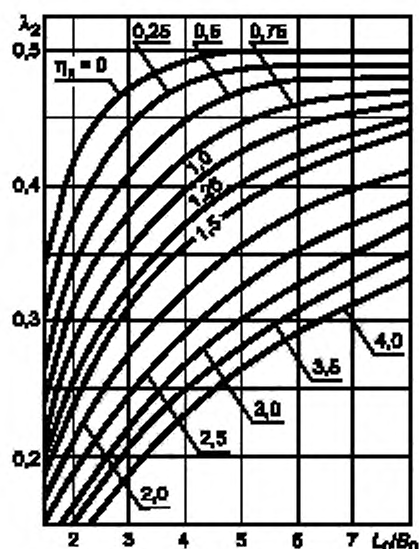
Рисунок И.2 — График коэффициента \lambda_2
