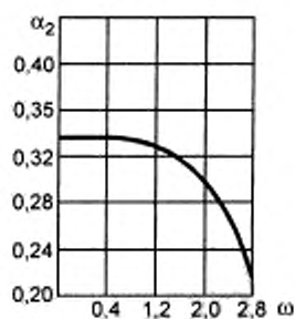
Рисунок И.4 — График коэффициента \alpha_2
