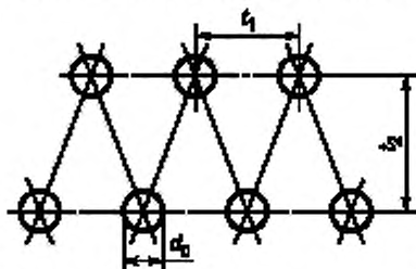
Рисунок Ж.2 — Расположение отверстий по вершинам треугольников
