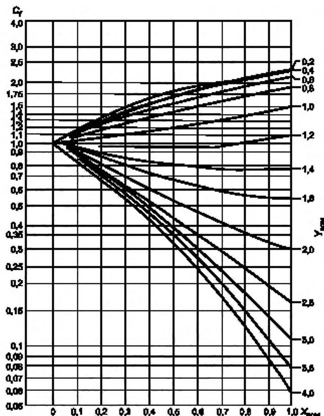
Рисунок 25 — Параметр жесткости компенсатора C_T
