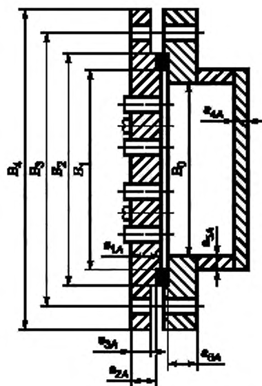
Рисунок 15 — Камера разъемной конструкции со сварной крышкой
