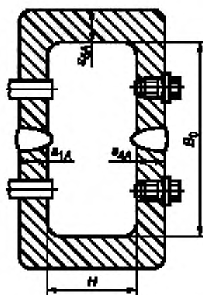
Рисунок 22 — Штампованная камера без перегородок
