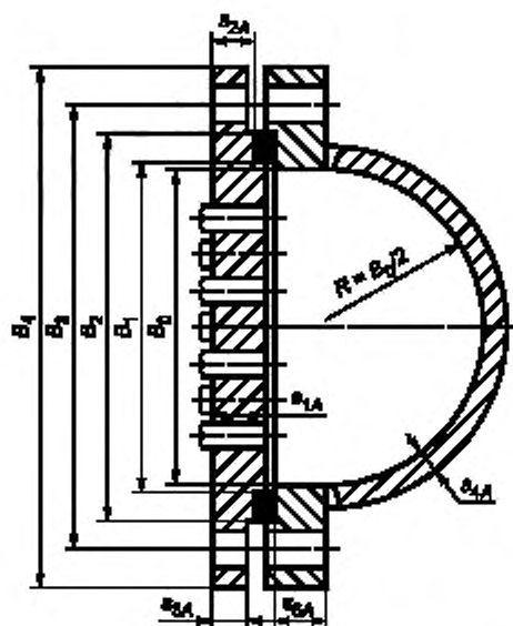
Рисунок 18 — Камера разъемной конструкции со сварной полусилиндрической крышкой
