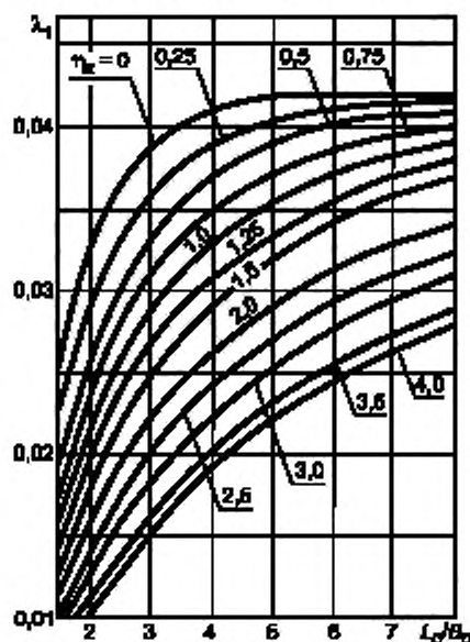
Рисунок И.1 — График коэффициента \lambda_1
