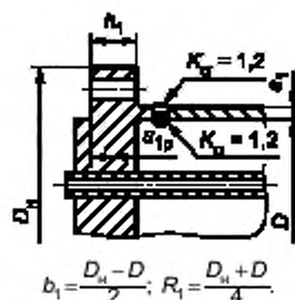
Рисунок 8 — решетка, приваренная встык к обечайке кожуха
