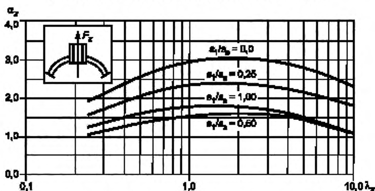
Рисунок 8 — Коэффициенты концентрации в месте пересечения проходящего штуцера со сферической оболочкой при осевом усилии на штуцер
