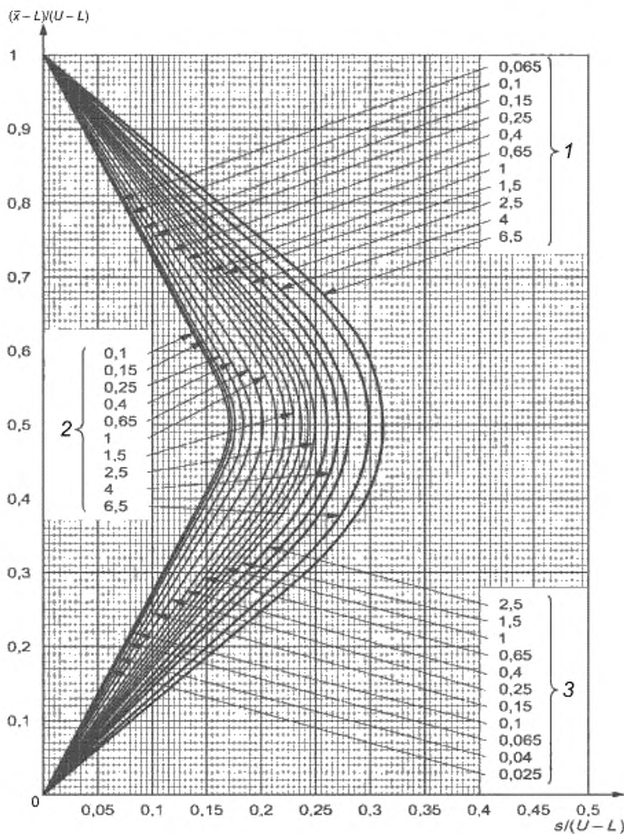
Рисунок 27 — График s-L. Приемочные кривые для объединенного контроля с двумя пределами поля допуска и общим AQL. «s» метод. Код объема выборки L (объем выборки 70) (для ослабленного контроля код объема выборки N)
