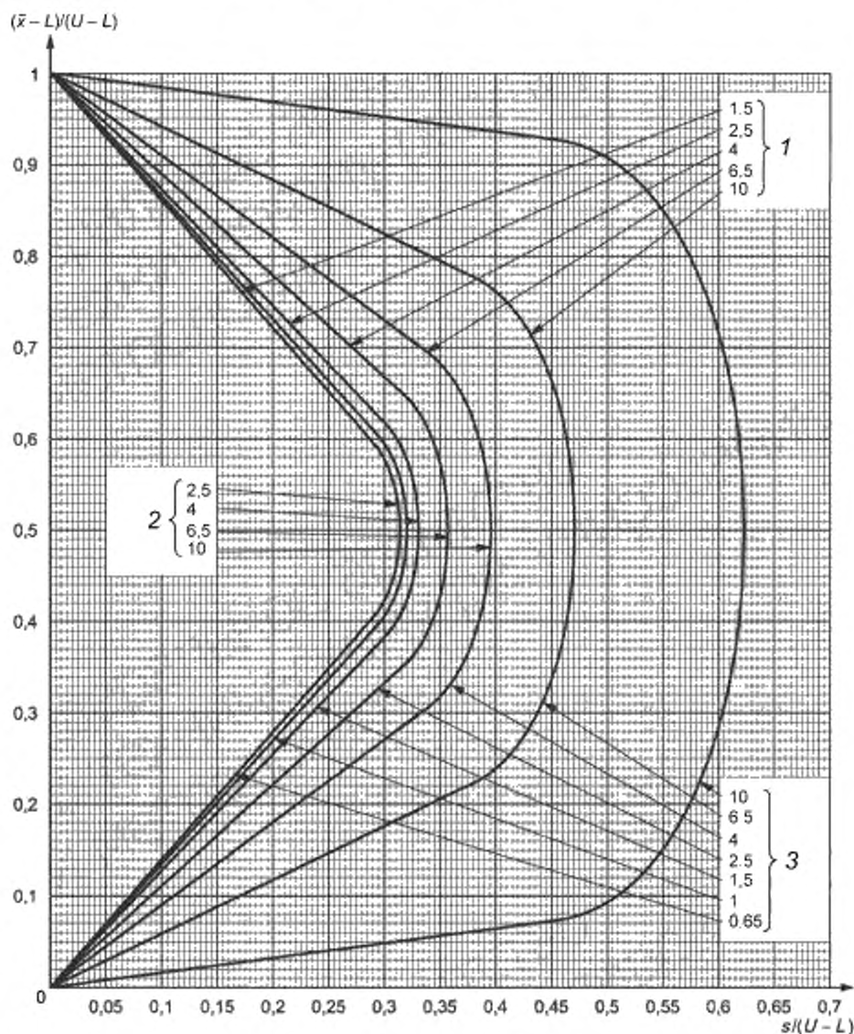
Рисунок 20 — График s-D. Приемочные кривые для объединенного контроля с двумя пределами поля допуска и общим AQL. «s» метод. Код объема выборки D (объем выборки B) (для ослабленного контроля код объема выборки F)
