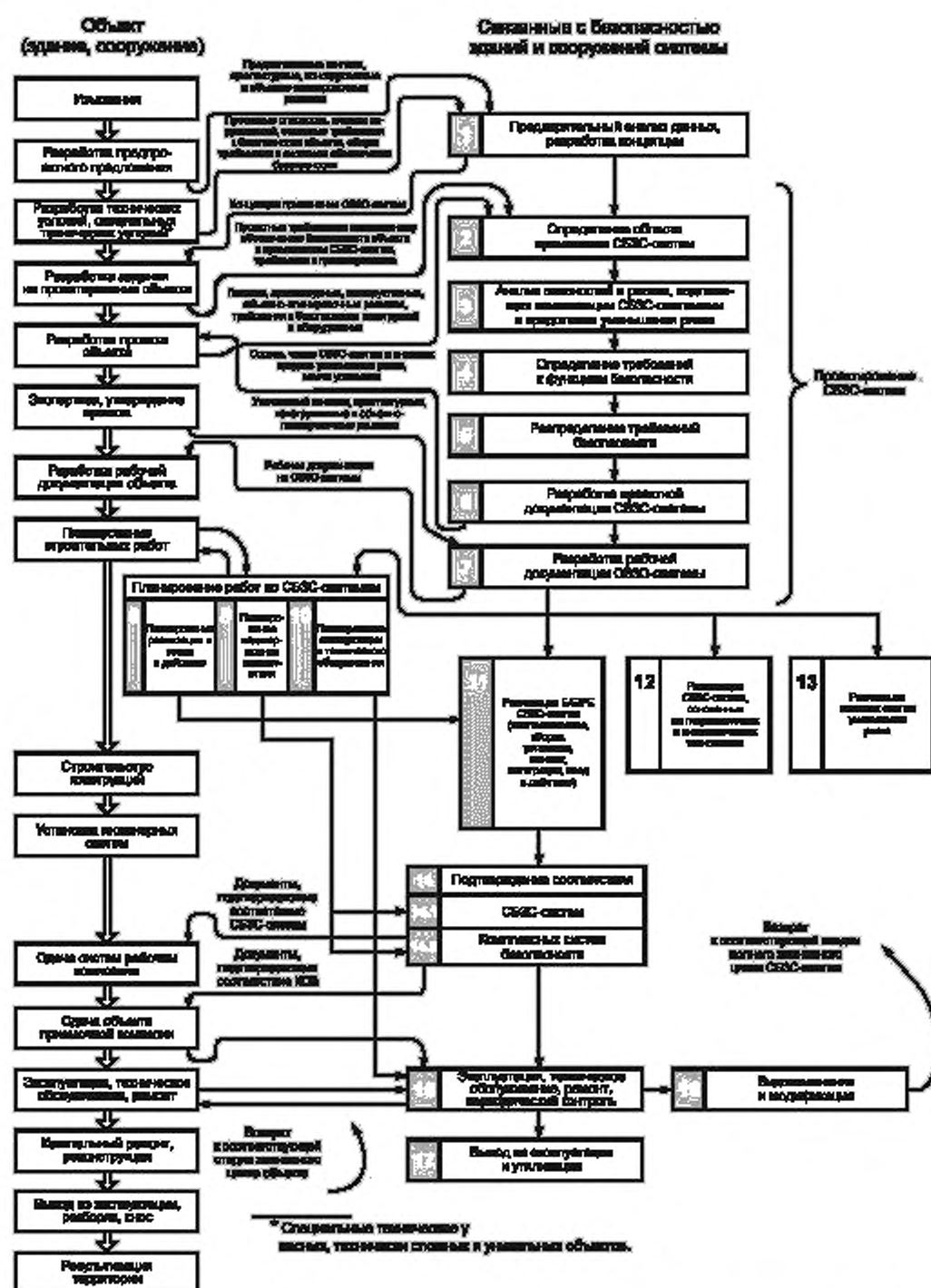
Рисунок 1 — Базовая структура полного жизненного цикла E/E/PE CBZC-систем и жизненного цикла зданий и сооружений
