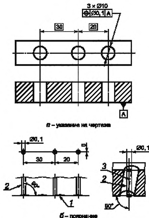
1 – моделированная база A; 2 — поле допуска; 3 — выявленная средняя линия отверстия
