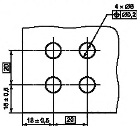
Рисунок А.1 — Указание на чертеже
