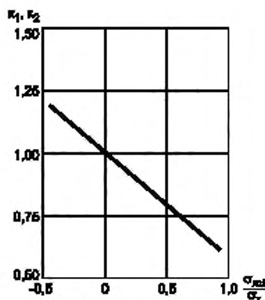
Рисунок А.1 — Диаграмма зависимости коэффициентов k_1, k_2 от значения относительной величины суммарных средних напряжений \frac{\sigma_{m1}}{\sigma_T}
