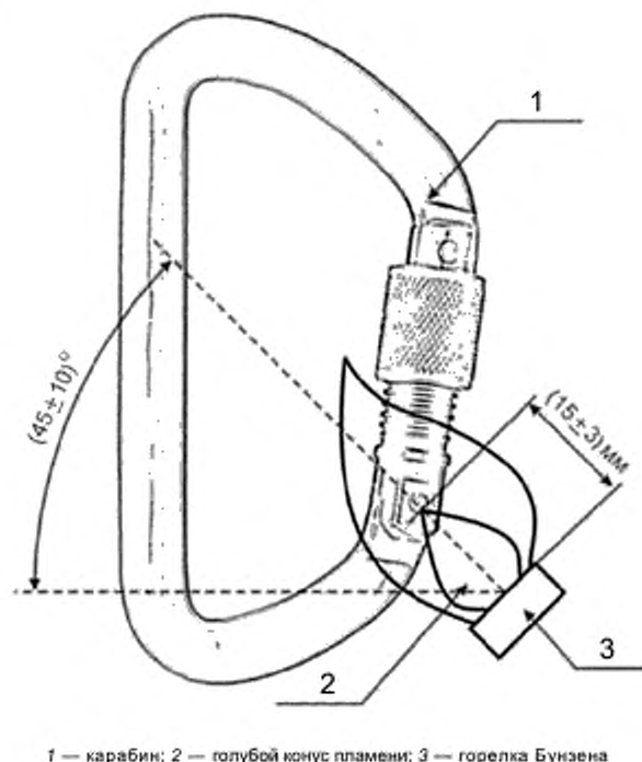
1 — карабин; 2 — голубой конус пламени; 3 — горелка Бунзена
