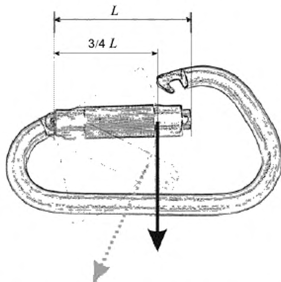
Рисунок 2 — Схема испытания усилия раскрытия затвора карабина
