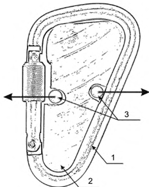
1 — карабин; 2 — оправка; 3 — силовые скобы
