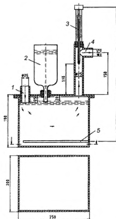
Рисунок В.2 — Схема холодильника
