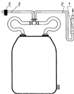
1 — ротаметр; 2 — соединительные трубки; 3 — зажим
