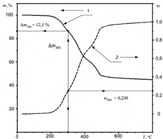
Рисунок В.6 — Схема определения идентификационных характеристик при фиксированной температуре T = 300^{\circ}\text{C}
