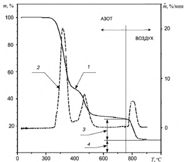
Рисунок В.4 — Схема определения коксового и зольного остатков по термогравиметрической кривой (в координатах «сигнал — температура»)
