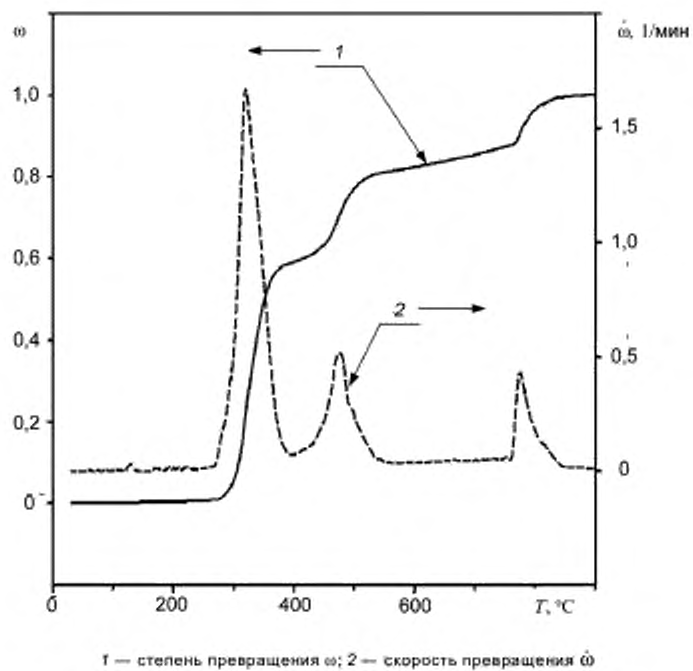
Рисунок А.2.1 — Характерные термовалитические кривые образца материала
