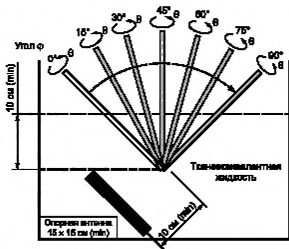
\theta — угол поворота зонда вокруг своей оси; \varphi — угол наклона оси зонда
