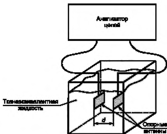
Рисунок В.2 — Схема установки для измерения коэффициента усиления антенны
