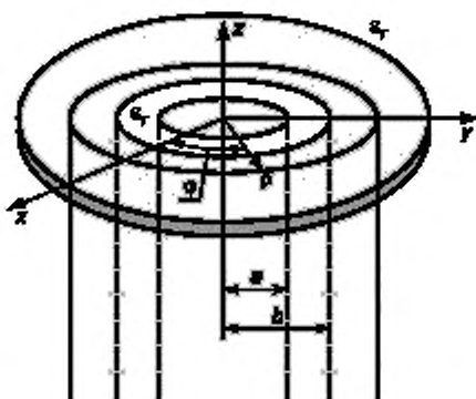
Рисунок Ж.2 — Коаксиальный зонд с открытым концом с внутренним и внешним радиусами a и b соответственно
