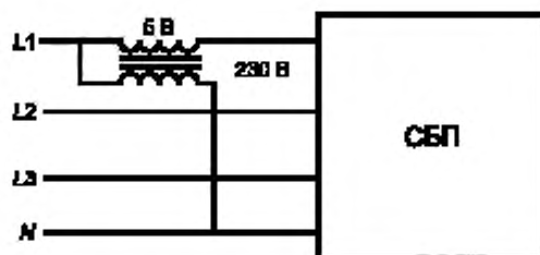
Рисунок D.1 — Амплитудная несимметрия
