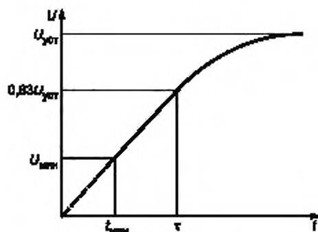
Рисунок 2 — Кривая натекания
