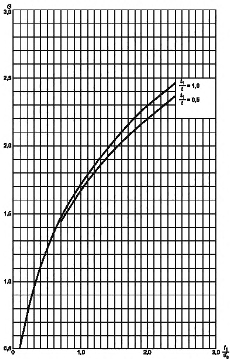
Рисунок 2 — Геометрический фактор G для двухжильного кабеля с поясной изоляцией и круглыми жилами (см. 2.1.2.1)
