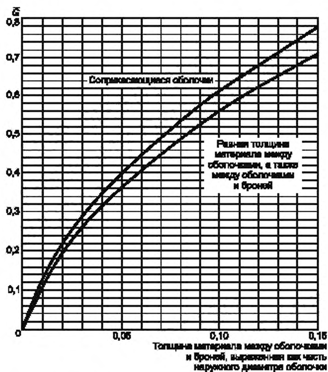
Рисунок 6 — Геометрический фактор \bar{G} для определения тепловых сопротивлений заполняющего материала, находящегося между оболочками и броней кабелей типов SL и SA (см. 2.1.2.2)
