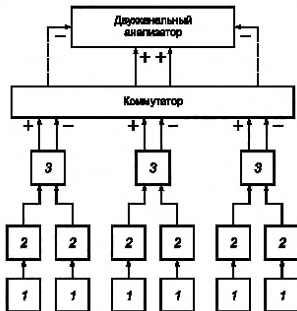
1 — датчик ускорения; 2 — предварительный усилитель (усилитель заряда); 3 — сумматор
