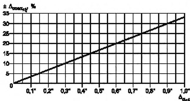
Рисунок В.1 — Зависимость максимальной погрешности \pm \Delta_{\cos \alpha_{c\phi}} от угла сдвига фаз между измерительными каналами силы и скорости при \alpha_{Fq \max} = 87^\circ
