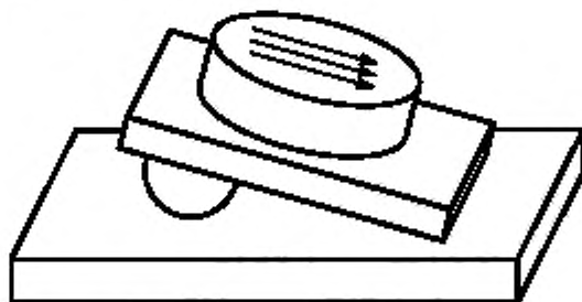
Рисунок 3 — Пример наклонной оптической пластины и схемы измерений
