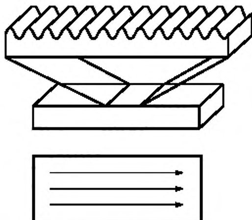
Рисунок 2 — Пример эталона шага неровностей (тип С)
