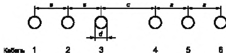
Рисунок 1 — Расположение кабелей
