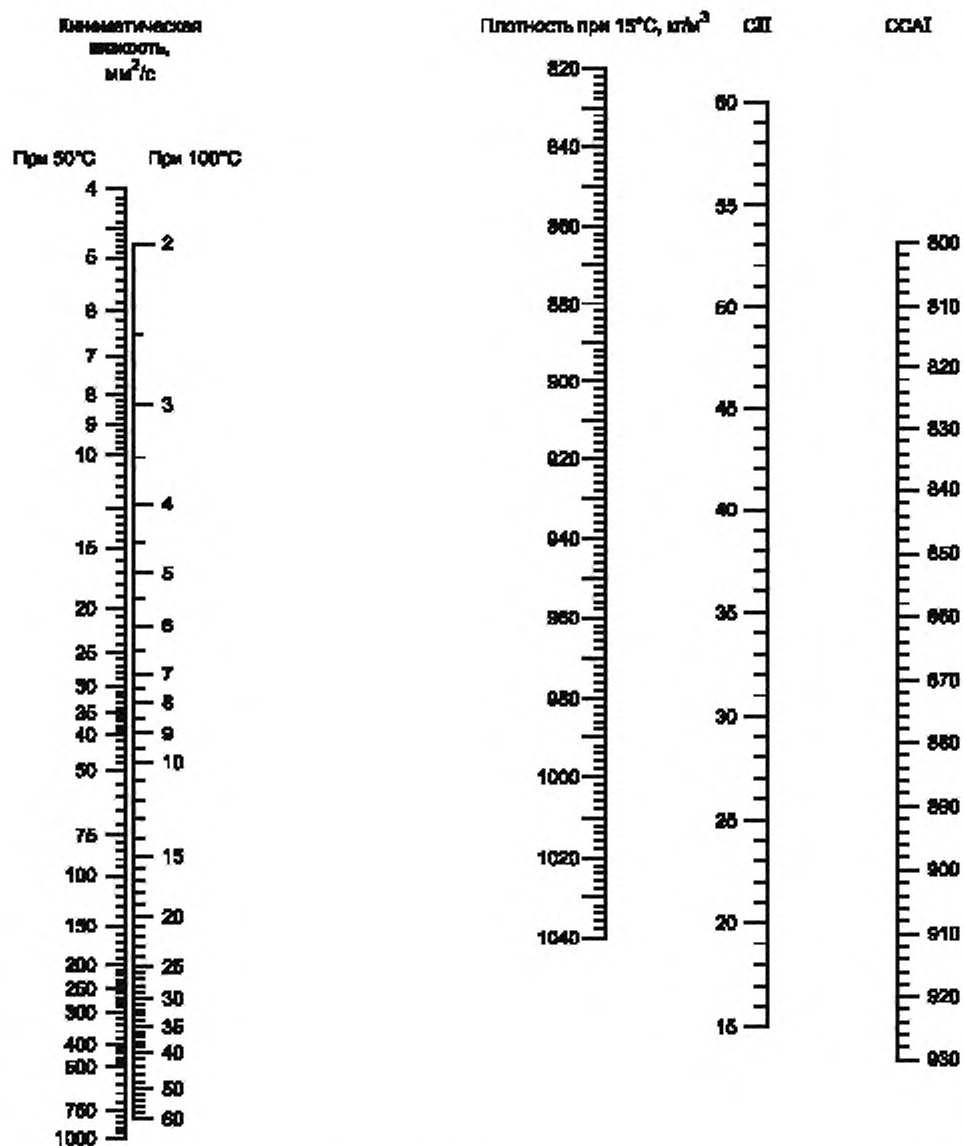
Рисунок А.1 — Номограмма для определения индекса воспламеняемости СИ и индекса ароматичности ССАИ
