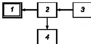
1 — испытуемое оборудование; 2 — делитель мощности; 3 — высокочастотный генератор сигналов; 4 — анализатор спектра
