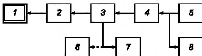
Рисунок 3 — Схема подключения оборудования при проверке пределов и определении погрешности измерения ширины полосы частот до 300 кГц
