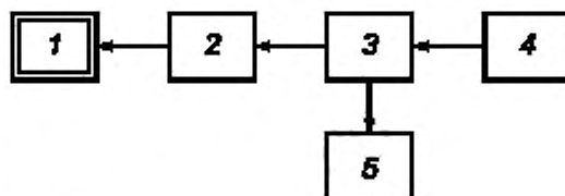
Рисунок 5 — Схема подключения оборудования при определении пределов и погрешности измерения коэффициента АМ
