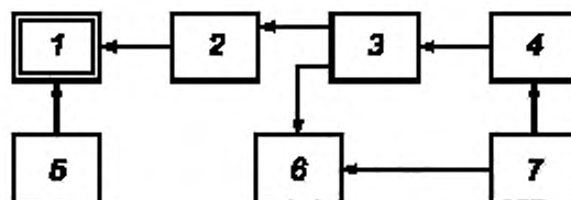
Рисунок 1 — Схема подключения оборудования при определении диапазона рабочих частот и погрешности измерения частоты немодулированных сигналов
