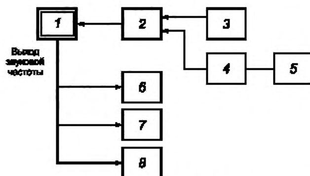
1 — испытываемое оборудование; 2 — сумматор сигналов; 3 — генератор А; 4 — ФНЧ (при необходимости); 5 — генератор Б; 6 — эквивалент нагрузки; 7 — вольтметр; 8 — измеритель нелинейных искажений
