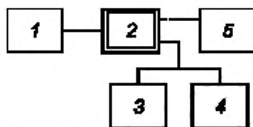
1 — высокочастотный генератор сигналов; 2 — испытуемое оборудование; 3 — вольтметр переменного тока; 4 — эквивалент нагрузки; 5 — анализатор спектра
