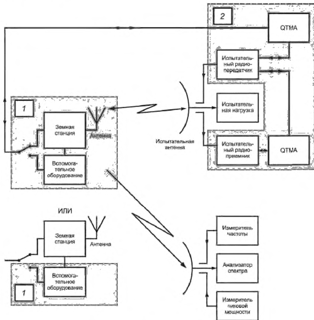
Рисунок 1 — Конфигурация оборудования при испытаниях
