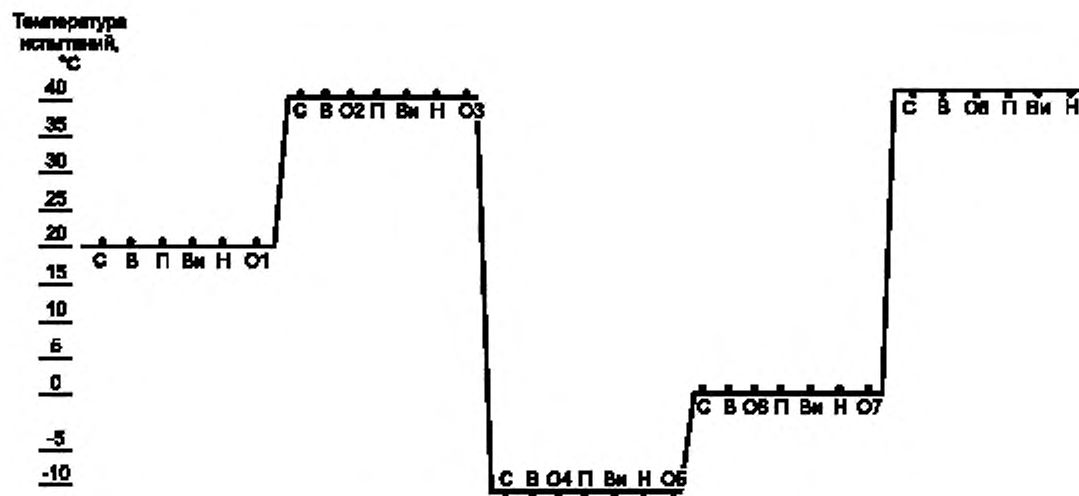
Рисунок 11 — Предлагаемая последовательность испытаний по А.5.3.1, совмещенных с А.5.3.2 (температурные испытания в диапазоне от минус 10 °С до плюс 40 °С)
