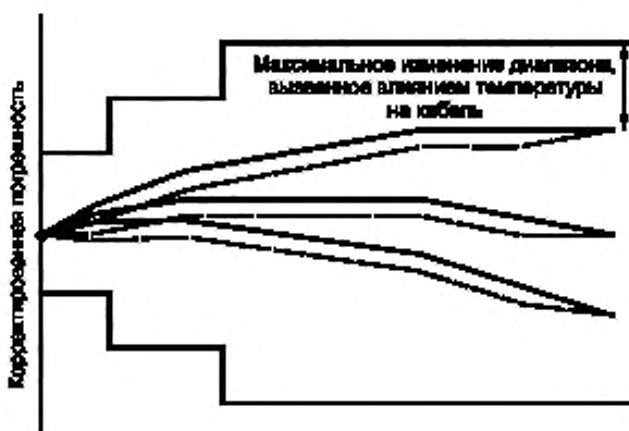
Рисунок 12 — Изменение диапазона из-за влияния температуры на кабель
