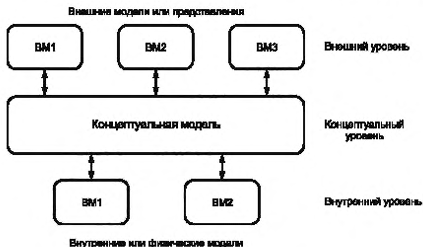
Рисунок 3 — Трехуровневая архитектура
