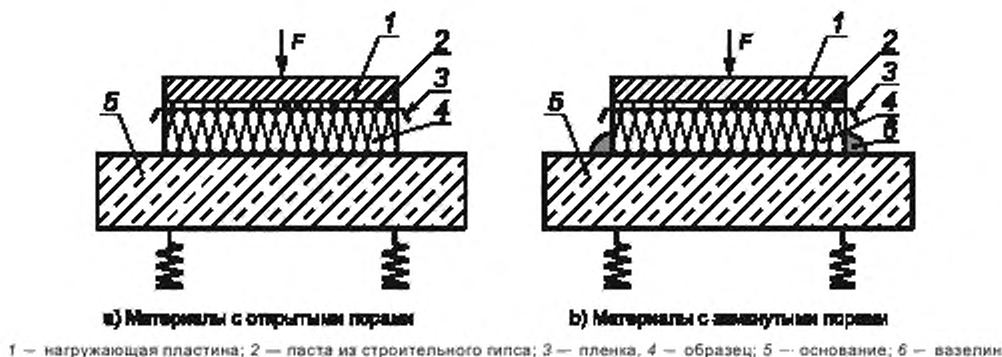
Рисунок 3 — Возбуждение нагружающей пластины. Измерение вибрации нагружающей пластины и основания
