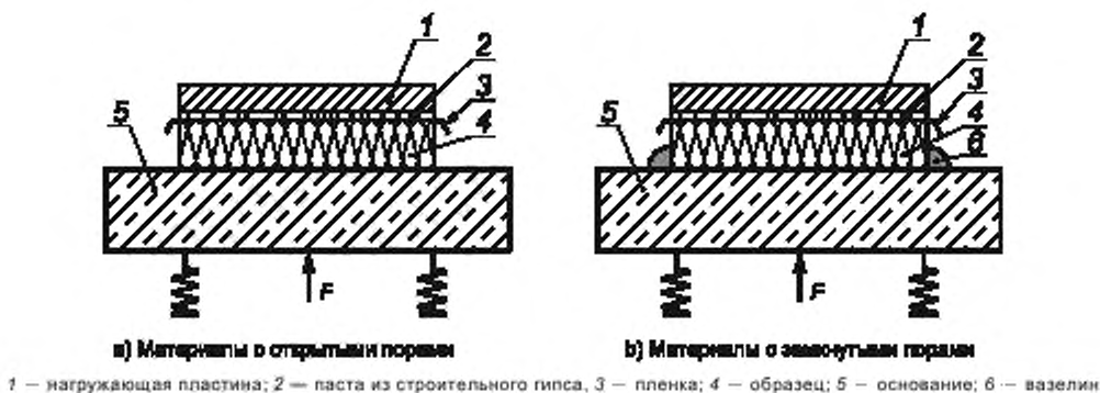
Рисунок 2 — Возбуждение нагружающей пластины. Измерение вибрации нагружающей пластины и основания
