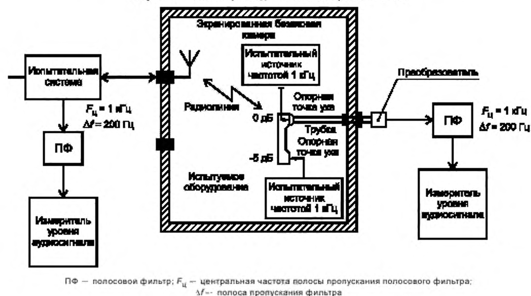
Рисунок 2 — Схема установки опорного уровня аудиосигнала при испытаниях
