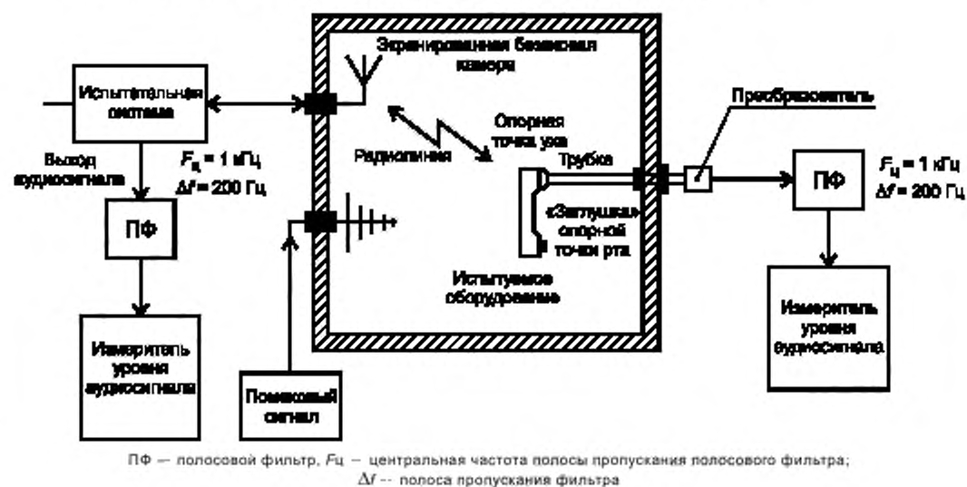
Рисунок 1 — Схема прохождения сигнала при испытаниях
