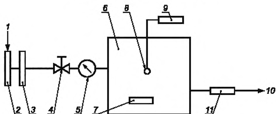
Схема установки с испытательной камерой
