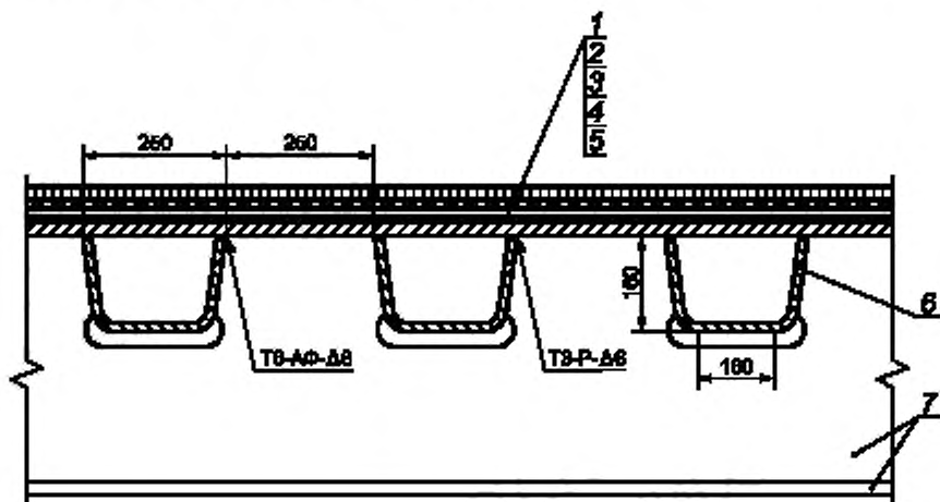
1, 2, 3 — система тонкослойного покрытия; 4 — слой заводской грунтотки; 5 — настильный лист ортотропной плиты; 6 — продольное ребро; 7 — стенка и пояс поперечной балки
