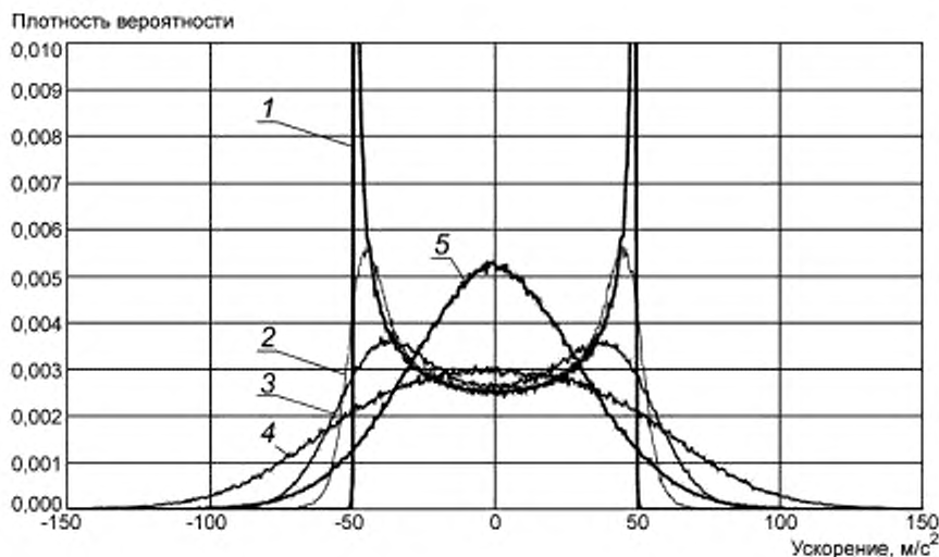
1 — чисто гармонический сигнал; 2 — гармонический и случайный (СПУ — 0,1 \text{ м}^2/\text{с}^3 ) сигналы; 3 — гармонический и случайный (СПУ — 1 \text{ м}^2/\text{с}^3 ) сигналы; 4 — гармонический и случайный (СПУ — 5 \text{ м}^2/\text{с}^3 ) сигналы; 5 — чисто случайный сигнал (СПУ — 5 \text{ м}^2/\text{с}^3 )
