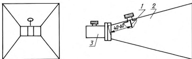
Приемопередающая антенна
