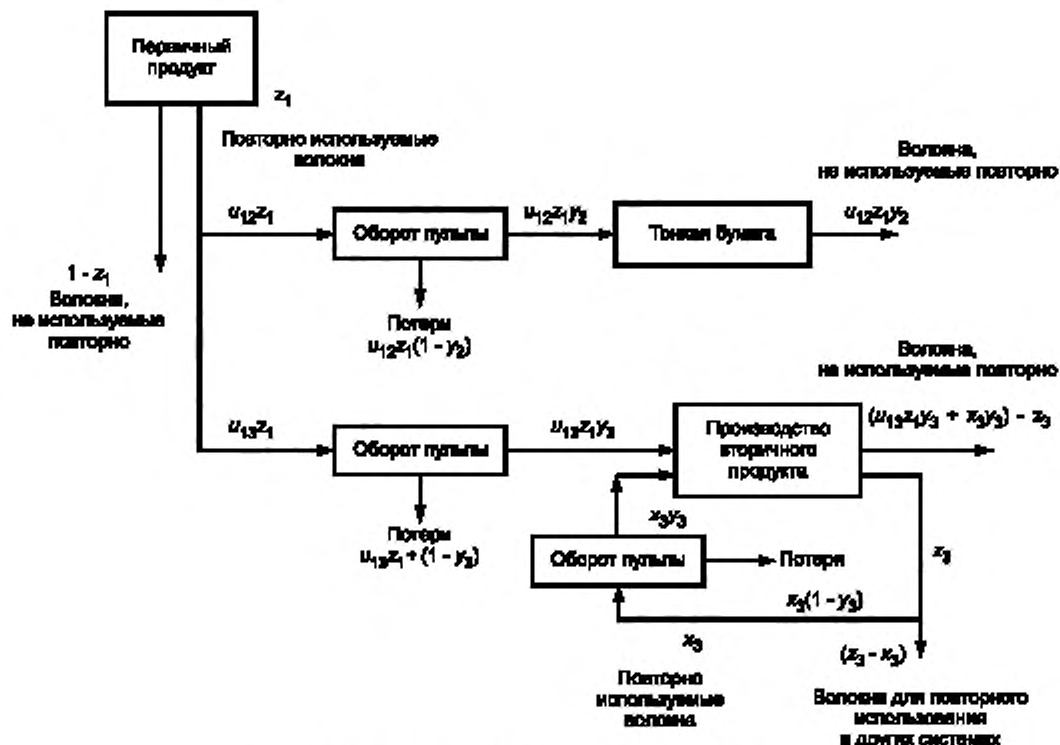
Рисунок 21 — Разные применения отходов и извлеченного КВРВ
