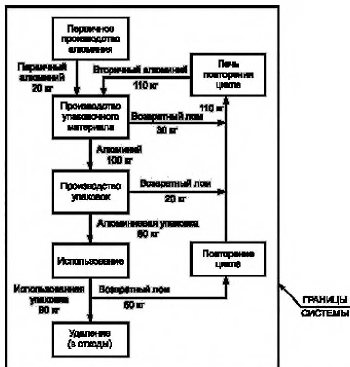
Рисунок 18 — Модель повторения цикла для алюминиевой упаковки с коррективным разделением технологического процесса выпуска специальной продукции
