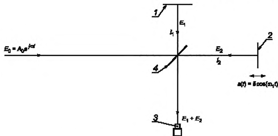
1 — зеркало 1; 2 — зеркало 2; 3 — фотодетектор; 4 — разделитель луча
