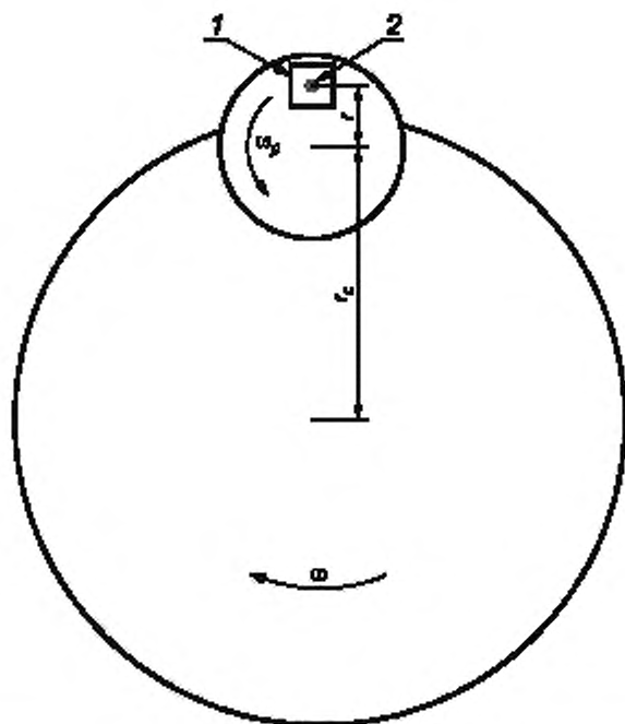
1 — испытуемый преобразователь; 2 — центр тяжести сейсмической массы преобразователя
