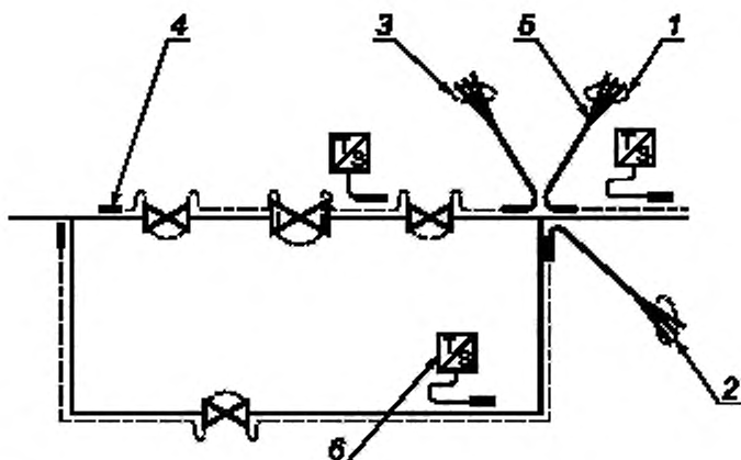
Рисунок 5 — Пример обогреваемого резервуара
