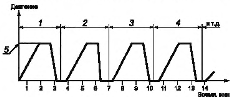
1 — отсек 1, 2 — отсек 2; 3 — отсек 1; 4 — отсек 2; 5 — расчетное рабочее давление
