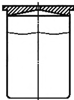
Рисунок 1 — Металлический пикнометр
