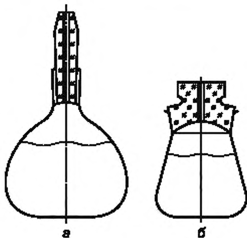
Рисунок 2 — Стекланный пикнометр
